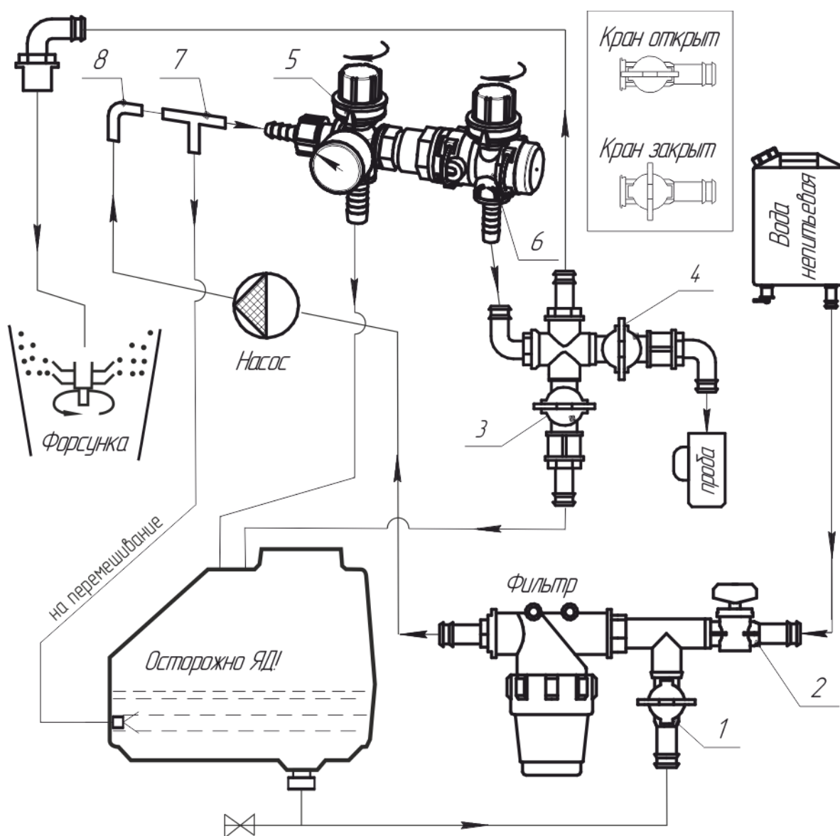
Рис. 7. Схема гидравлическая.
