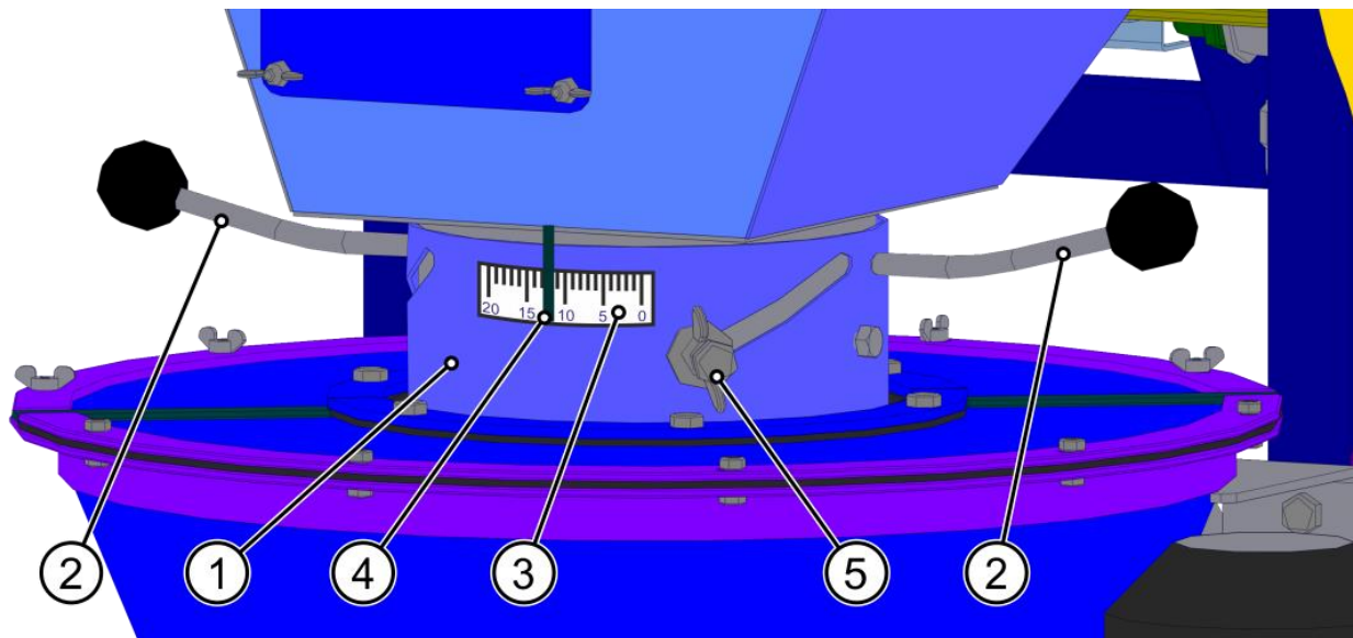
Рис. 6. Регулировка производительности по зерну.
