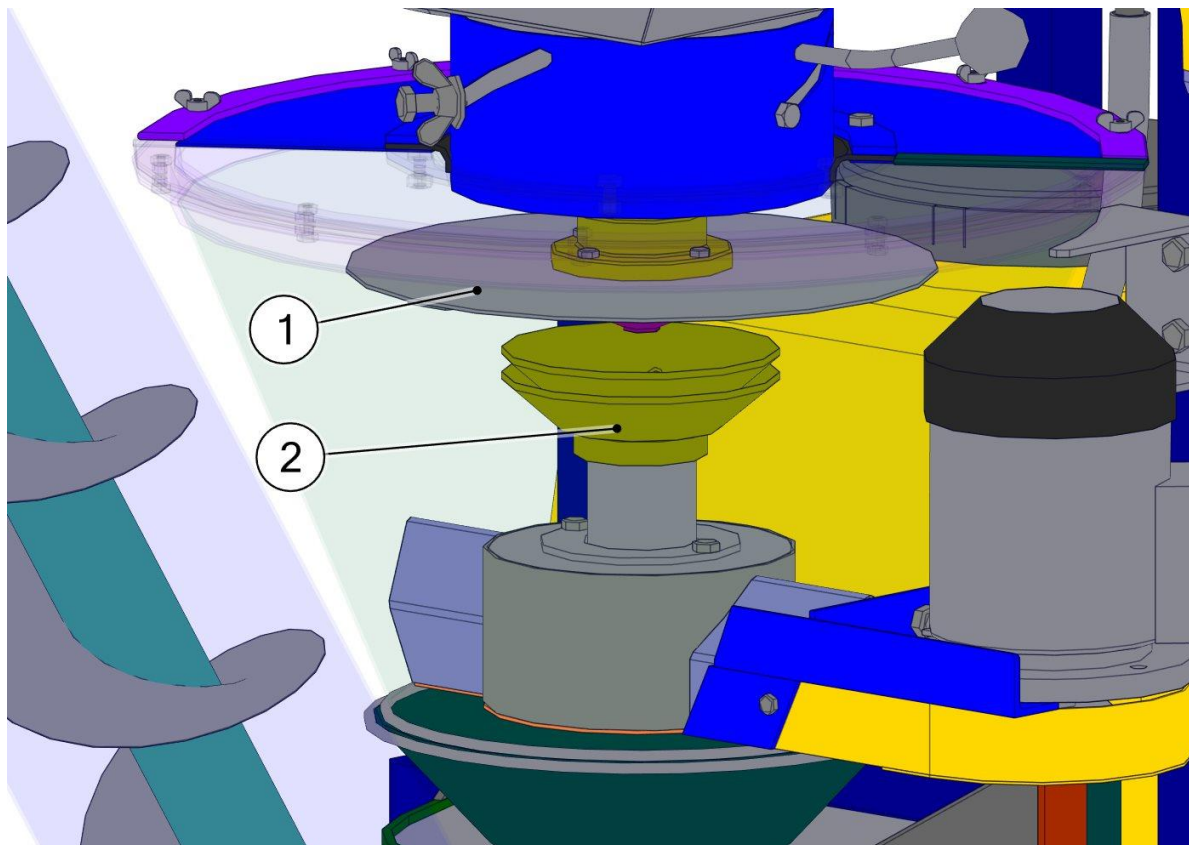
Рис. 4. Устройства, расположенные в камере протравливания.
