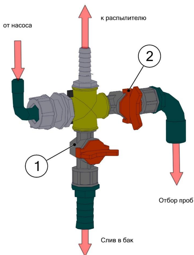
Рис. 5. Блок управления потоком жидкости.
