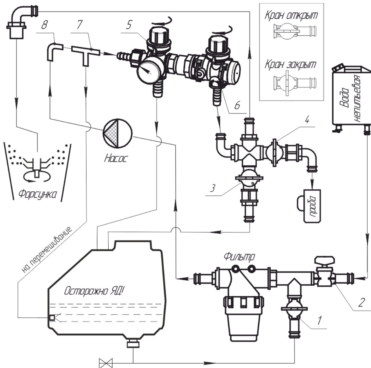
Рис. 7. Схема гидравлическая.
