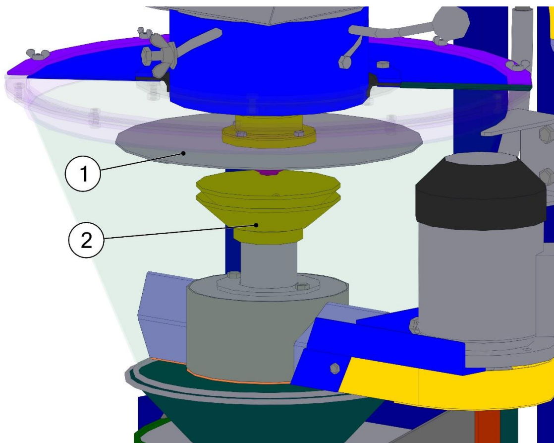
Рис. 4. Устройства, расположенные в камере протравливания.
