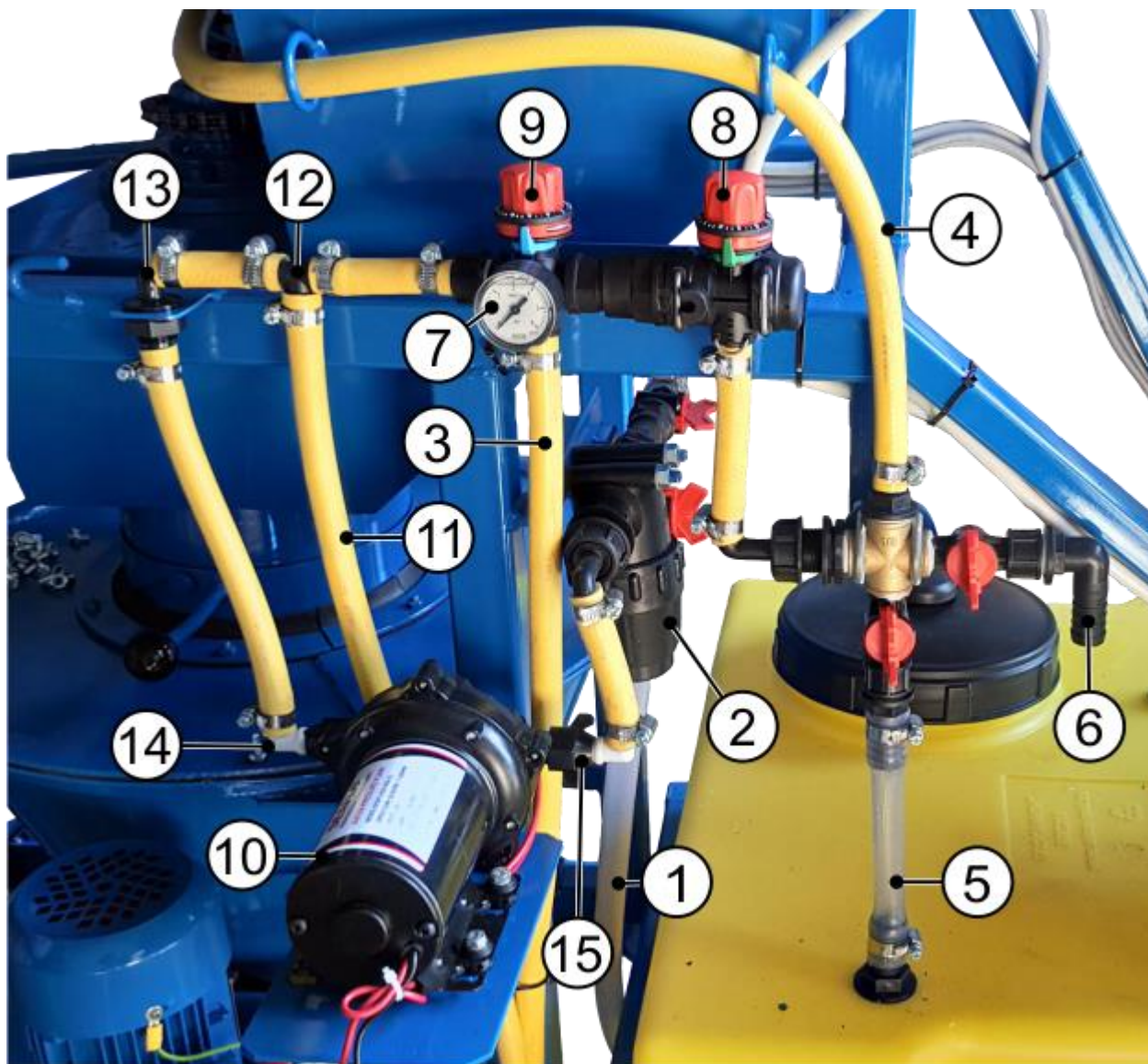
Рис. 8. Подключение насоса-дозатора.
