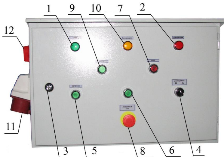
Рис. 3*. Пульт управления.
