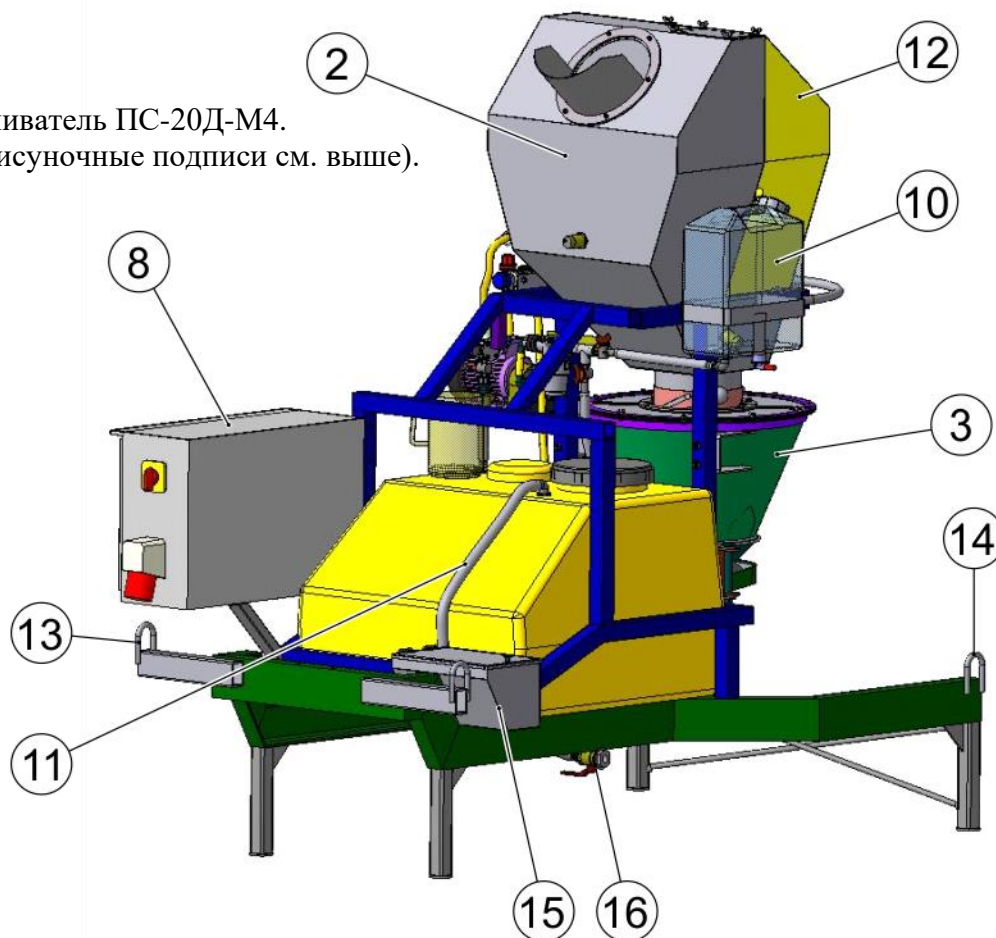
Рис. 1. Протравливатель ПС-20Д-М4. Вид справа.
